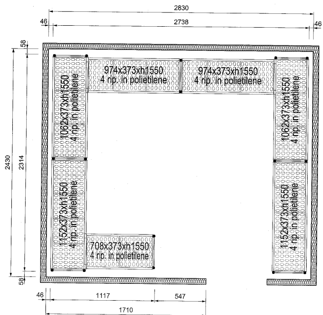
Boven aanzicht
